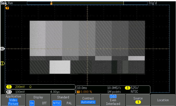
查看 NTSC 全彩条信号图像。视频图像模式包含了自动对比度和亮度设置以及手动控制。
