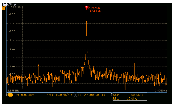
MDO3000 频域显示画面。
